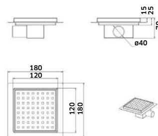
REF. AAM.201150. 78 Canelete de Duche Quadrado Grelha Perfurada
