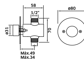
REF. TP0029. 271 Misturadora de Encastrar
