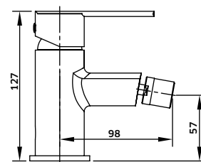
REF. 163019. 62 - Cromado Monocomando de Bidé
