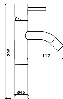
REF. 94017A. 123 - Cromado Monocomando de Lavatório Alto
