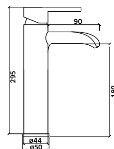
REF. 94617AC. 140 - Cromado Monocomando de Lavatório Cascata
