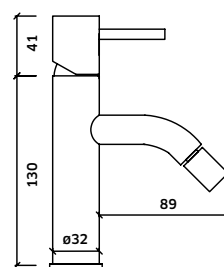
REF. 94119PR. 106 - Preto Monocomando de Bidé
