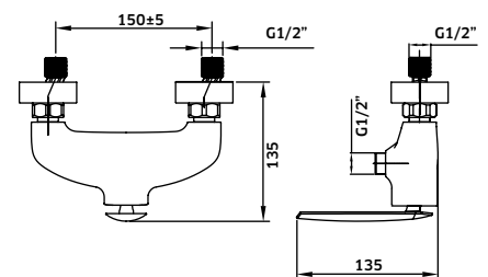
REF. 24323. 102 - Cromado Monocomando de Base de Chuveiro
