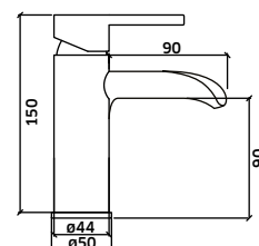
REF. 94617C. 97 - Cromado Monocomando de Lavatório Cascata
