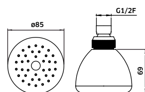
REF. CH0014F. 13 Chuveiro Parede 1 Função
