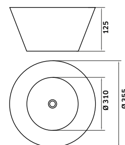
REF. LL031002. 135 - Preto Mate REF. LL031001. 90 - Branco Lavatório LENUS
