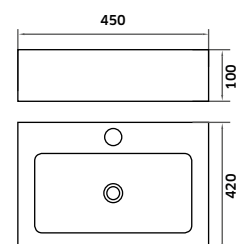
REF. LD0450001. 88 - Branco Lavatório DUATI
