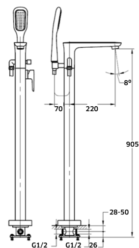
REF. 9030.790 Monocomando de Banheira ao Chão Quadrada
