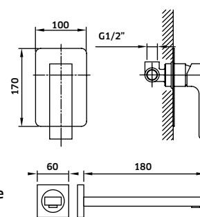
REF. 49530. 130 - Cromado Monocomando Lavatório à parede Bica Retangular
