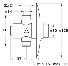
REF. TP0025. 74 Torneira de Chuveiro Encastrar
