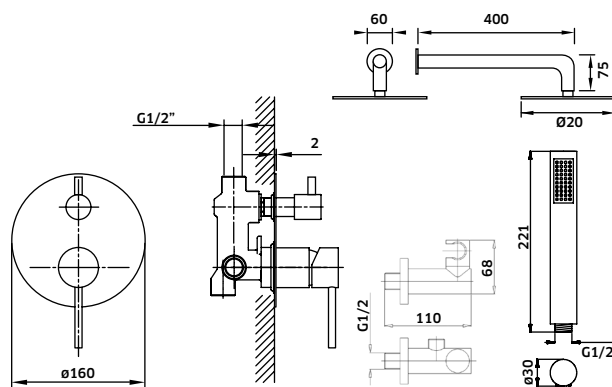
REF. 23426C. 189 Kit Duche 2 Vias Monoc. + Braço + Chuveiro + Suporte Chuveiro de Mão + Ligação
