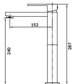
REF. 49517A. 115 - Cromado Monocomando de Lavatório Alto
