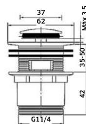
REF. 5011B. 11 Válvula clic-clac Bidê Espelho Pequeno
