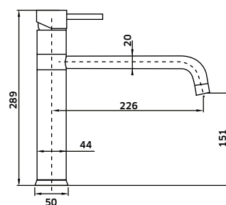
REF. 94026. 120 COSMOS Monocomando de Banca B.H.
