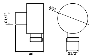
REF. 210031. 18 Tomada de água Cilíndrica
