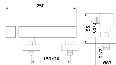
REF. 49023.85 - Cromado Monocomando de Base de Chuveiro
