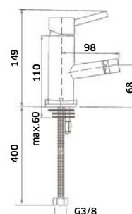
REF. 210019N. 49 - Cromado Monocomando de Bidê
