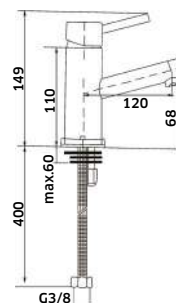
REF. 210017N. 49 - Cromado Monocomando de Lavatório
