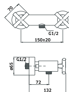
REF. 1903. 106 - Cromado Misturadora de Base de Chuveiro
