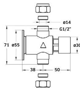
REF. TP0023. 55 Torneira de Chuveiro Externa
